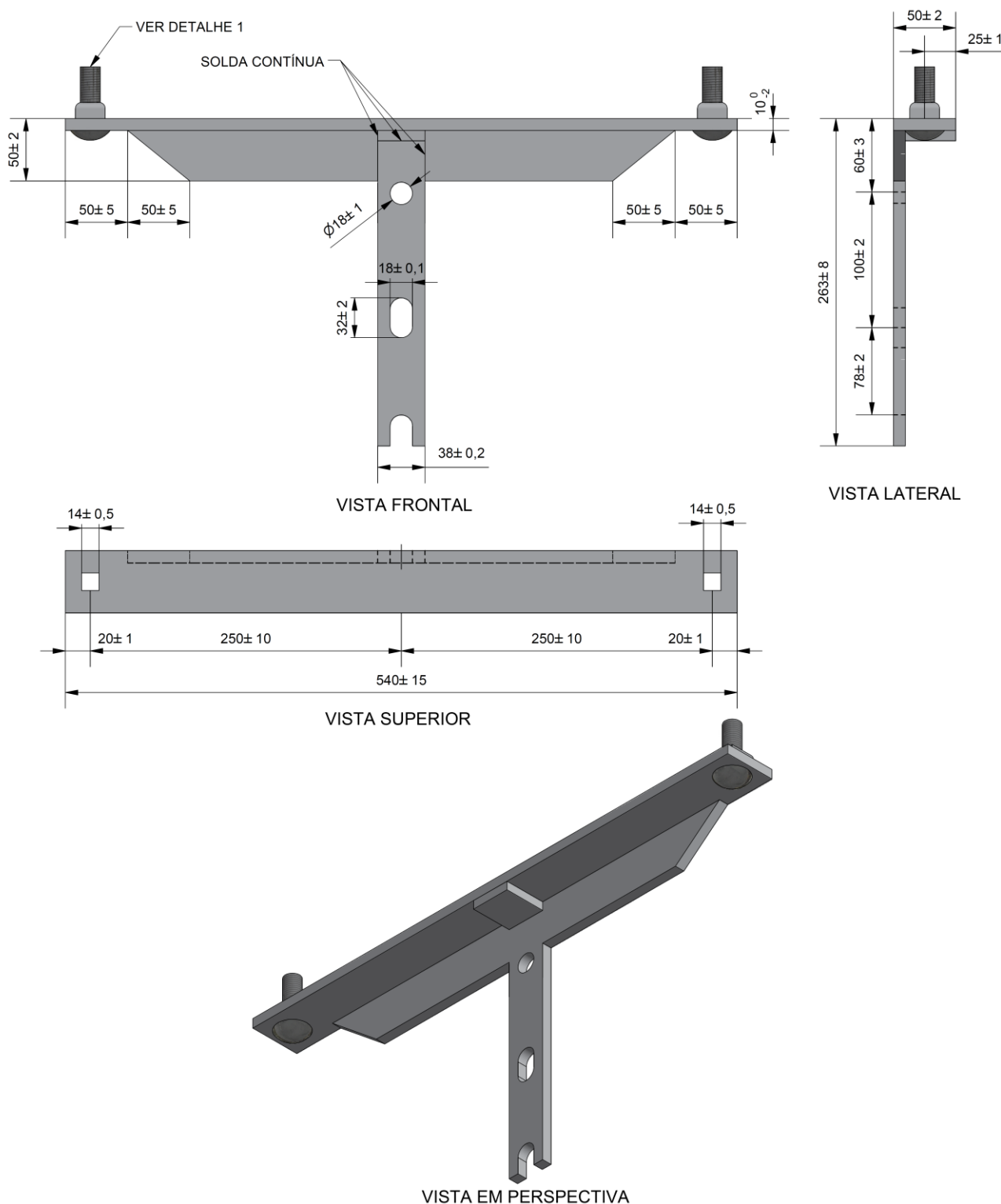
Figura 2 - Suporte T (TIPO 2)
