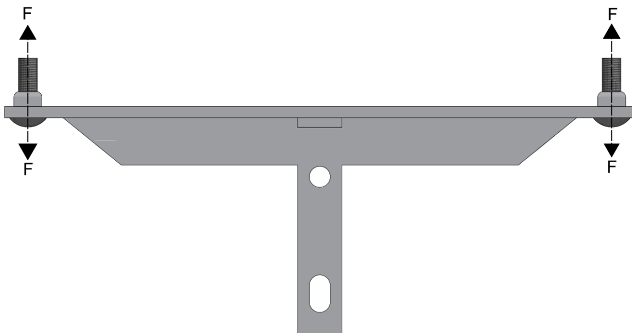
Figura 5 - Detalhe do ensaio
