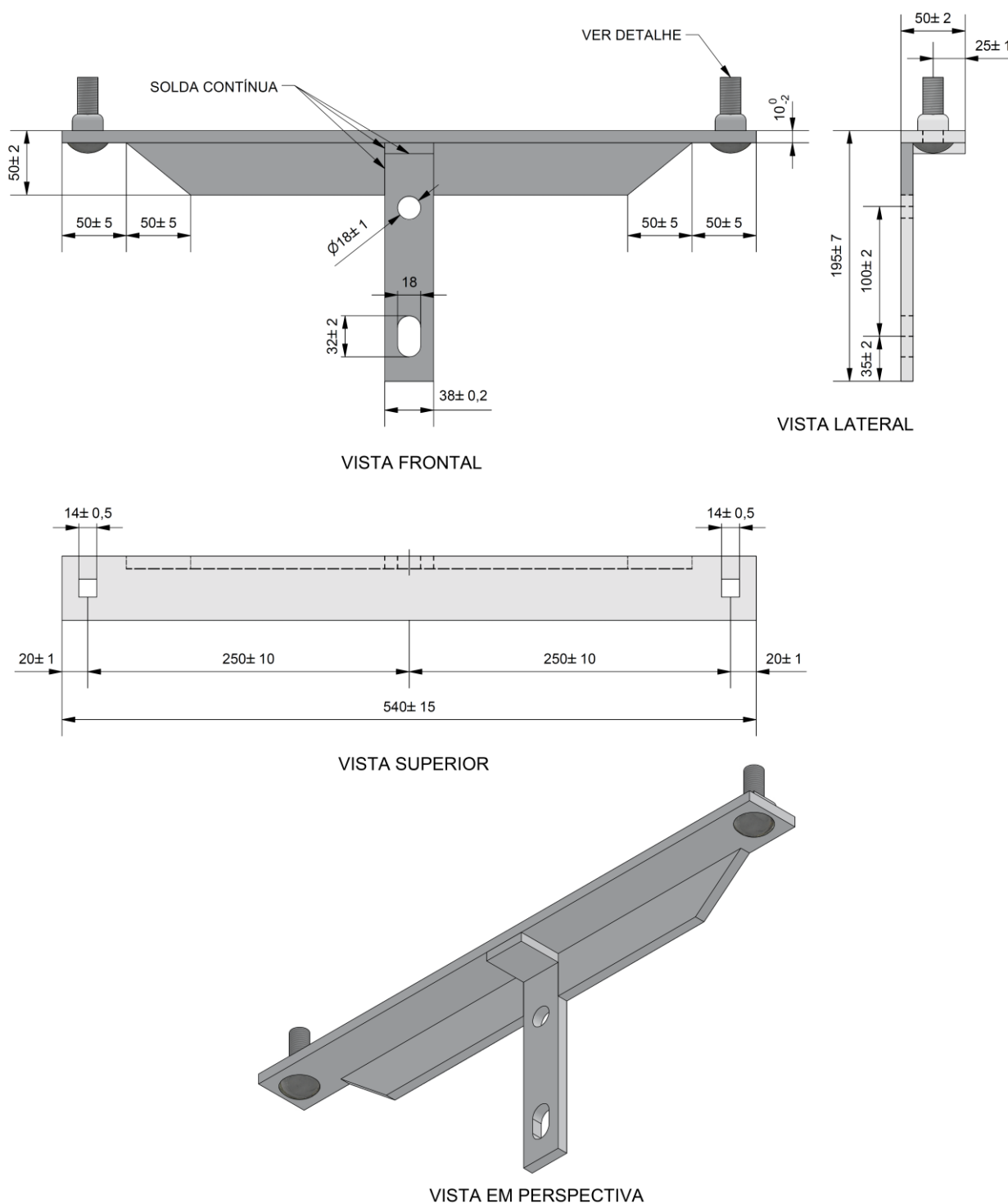
Figura 1 - Suporte T (TIPO 1)
