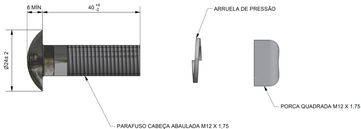
Figura 4 - Detalhe do Parafuso
